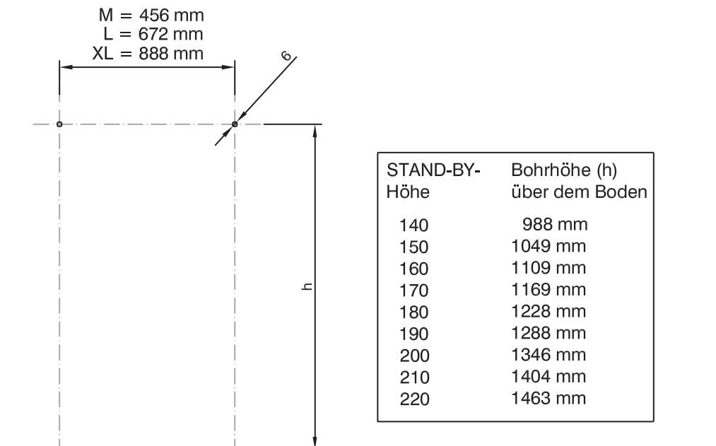
Zeichnung 2 Bohrpositionen
